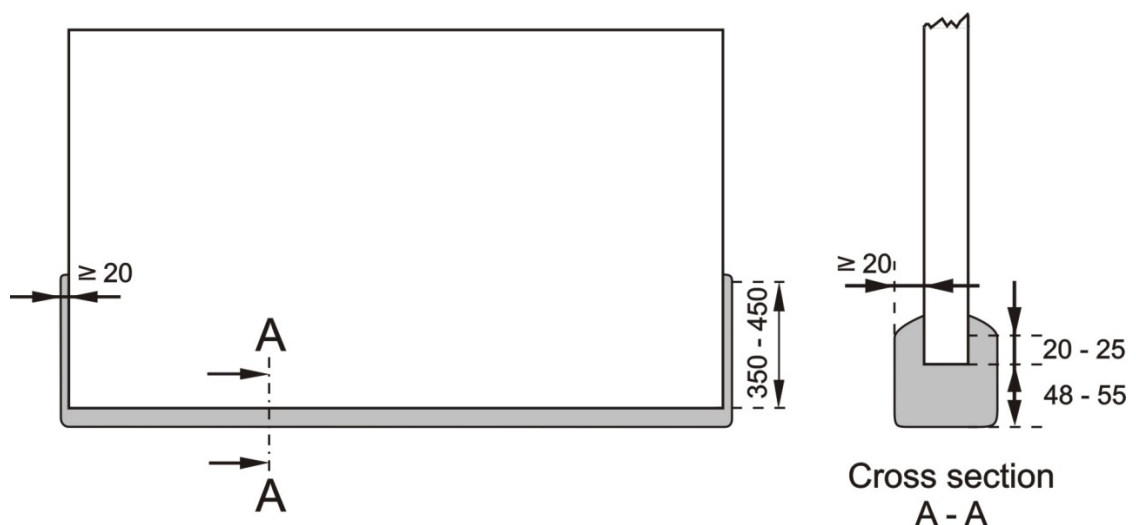
Рис. 7 Обивка щита
