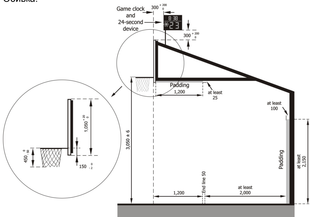
Рис. 1 Конструкция щита
