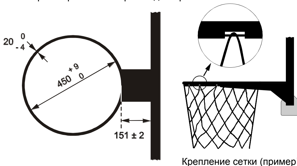
Рис. 4 Кольцо
